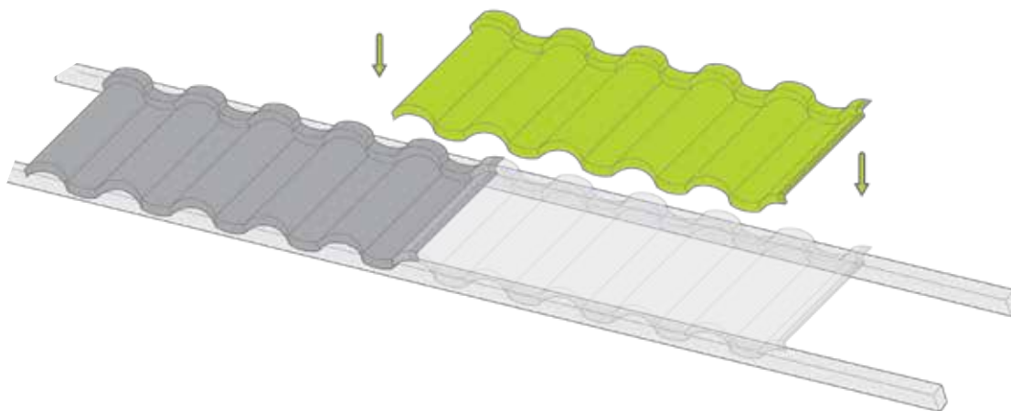
fig.34 NOVATIK ROMAN, SUPRAPUNERE LATERALĂ
