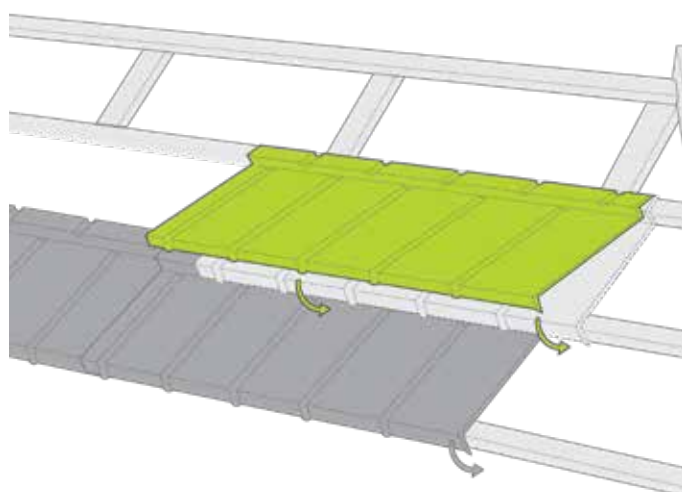
fig.20 SUPRAPUNEREA RÂNDURILOR
