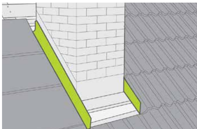
fig.55 ETANȘARE COȘ - PAS 2
