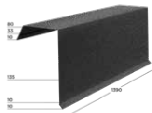
PAZIE
